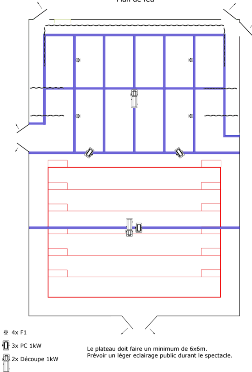
La Brigade des bonnes manières Plan de feu
